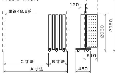
片開き収納時
