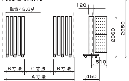
両開き収納時
